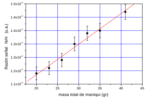
Figura 4. Relación señal N/H de maniquí.
