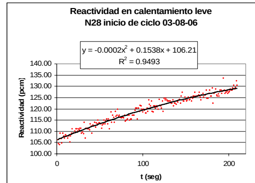
Figura 9. Valor de Reactividad ajustada en función del tiempo para la etapa de calentamiento leve.
