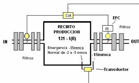
Figura 2. Sistema de control automático instalado en el recinto.
