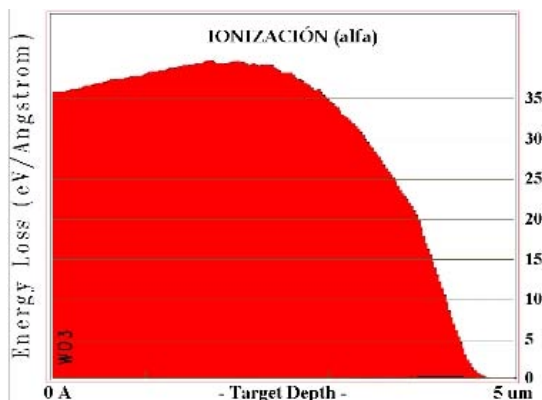
Figura 5. Distribución de la ionización ocasionada por las partículas alfa en \text{WO}_3 amorfo.
