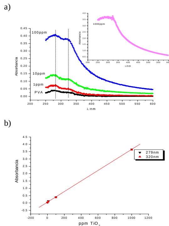
Figura 3. a) Espectros de absorción del \text{TiO}_2 en suspensión en PVA. b) Absorbancia vs concentración de \text{TiO}_2 a 279 y 320nm para mezclas de PVA- \text{TiO}_2 .
