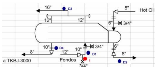
Figura 2. Arreglo experimental para la determinación de posibles pases de los fondos de la debutanizadora.
