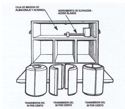
Figura 1. Conjunto de atenuadores.
