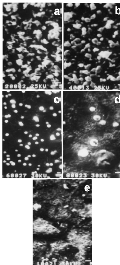
Figura 4. Micrografías SEM de recubrimientos obtenidas con soluciones precursoras con: (a) 20 % Zn y 80 % Sn, (b) 40 % Zn y 60 % Sn, (c) 60 % Zn y 40 % Sn, (d) 80 % Zn y 20 % Sn y (e) 100 % Zn.
