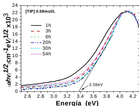
Figura 3. Variación de (\alpha h\nu)^{1/2} con respecto a la energía (h\nu) para diferentes tiempos de peptización.
