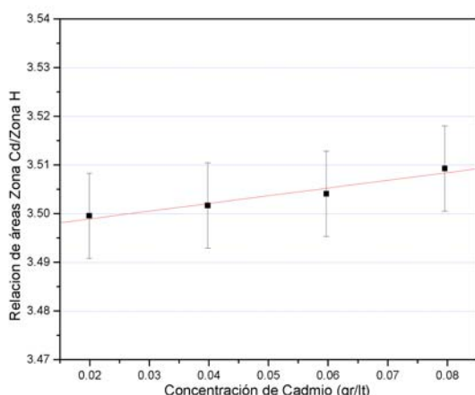
Figura 5. Razón de señales Cd/H, en relación de la concentración de cadmio para maniquí de calibración.
