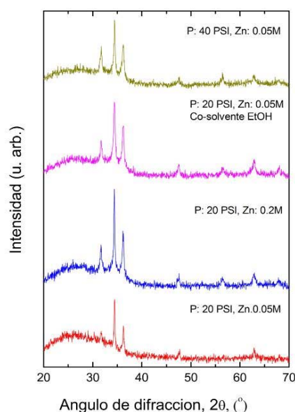
Figura 6. Difractogramas de rayos X de los recubrimientos obtenidos con soluciones precursoras con 75 % de Zn a diferentes condiciones de fabricación indicado en la figura.
