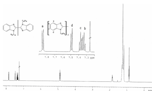
Figura 2. ^1\text{H} -RMN de 1,1'-bis(octadecil)-2,2'-bibenzimidazol.
