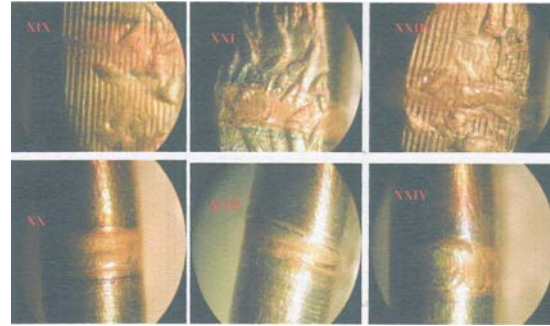
Figura 12. Ensayo de Impacto en la soldadura de los portafuentes
