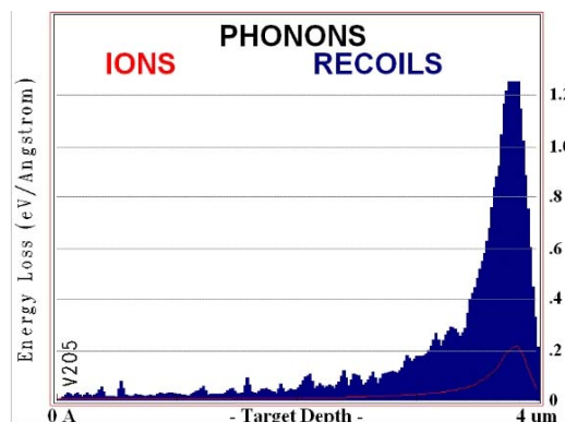
Figura 8. Distribución de la pérdida de energía a través de fonones de las partículas \alpha (área de rojo) y los recoils (área de azul) producidos dentro del \text{V}_2\text{O}_5
