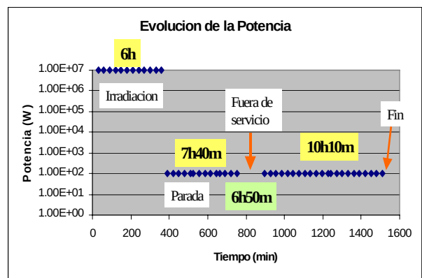
Figura 4. Potencia del reactor durante la experiencia. La operación duró 6 horas a 10 MW, la parada se extendió durante 7 horas con 40 minutos hasta que el veneno superó el exceso de reactividad. Transcurridos 6h50m se recuperó el crítico a 100W. La experiencia concluyó después de 24 horas con 50 minutos.
