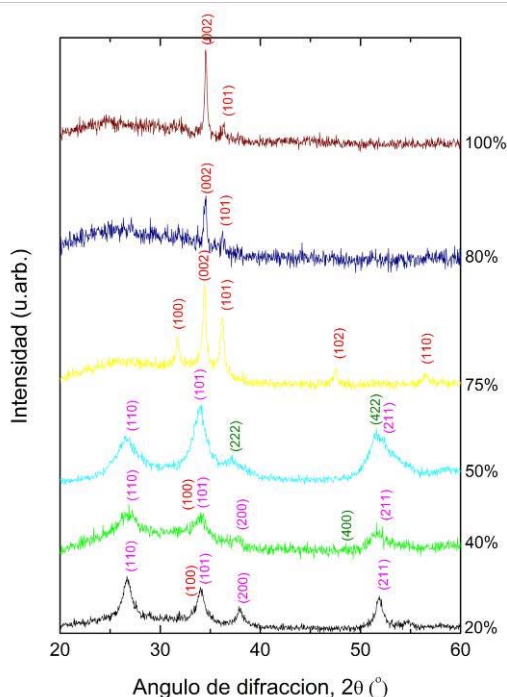
Figura 5. Difractogramas de rayos X de los recubrimientos obtenidos con soluciones precursoras con diferente contenido de Zn indicado en la figura.
