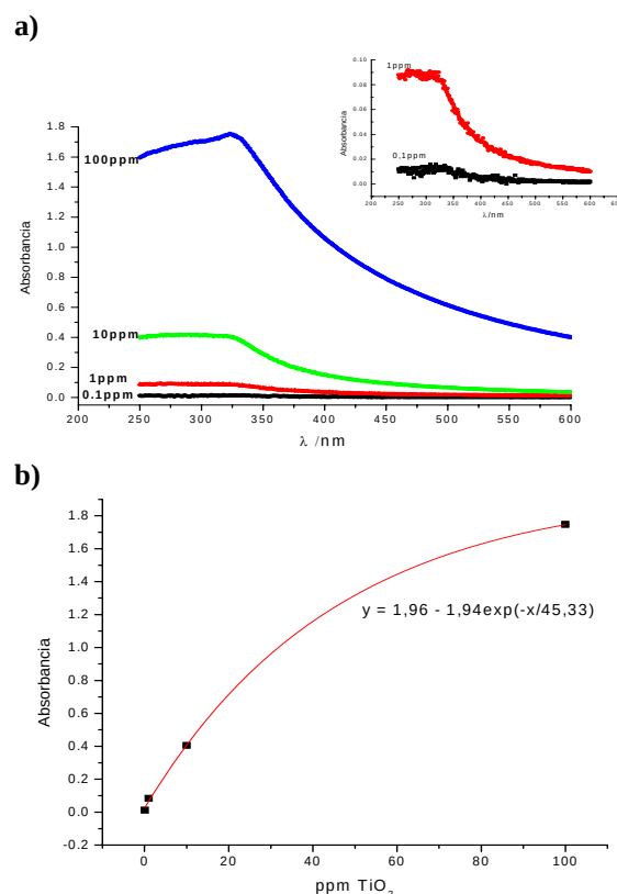
Figura 2. a) Espectros de absorción del \text{TiO}_2 en suspensión acuosa. b) Concentración vs absorbancia para las suspensiones acuosas de \text{TiO}_2 , a 325nm.
