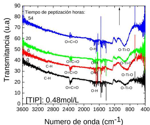
Figura 2. Espectros FTIR del \text{TiO}_2 a 1, 6, 20 y 54 horas de peptización depositados sobre sustrato conductor y deshidratados a 65° para una concentración de 0.48 mol/L
