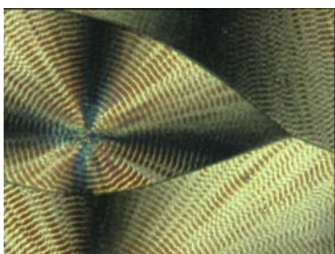
Figura 4. a) Textura esméctica C mostrada por el 2-octadecilbenzimidazol, y b) textura colestérica mostrada por el 1,1'-octadecil-2,2'-bibenzimidazol.
