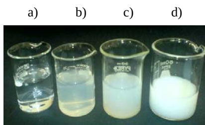
Figura 1. Mezclas de PVA- \text{TiO}_2 : a) solución acuosa de PVA, y suspensiones de \text{TiO}_2 , b) 10ppm, c) 100ppm y d) 1000ppm, en PVA estabilizadas por ultrasonido.
