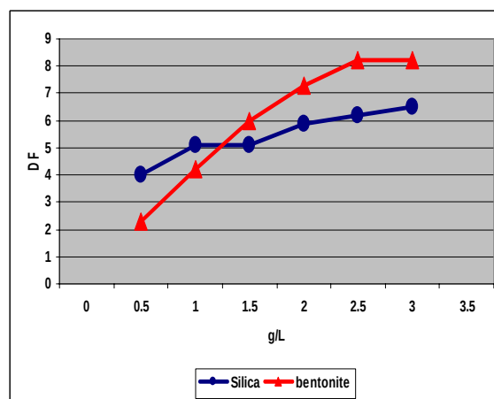
Figura 1. Variación del factor de descontaminación en función de la concentración de bentonita y silica gel.
