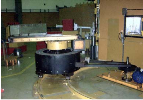
Figura 2. Instalación mecánica de ambos ejes.
