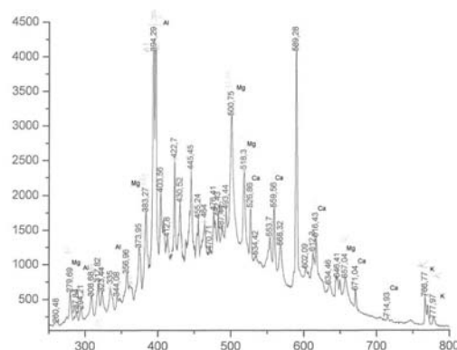
Figura 3. Espectro de cerámica Cajamarquilla y elementos identificados.
