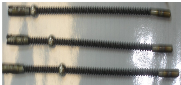
Figura 1. Portafuentes para discos de Ir-192.
