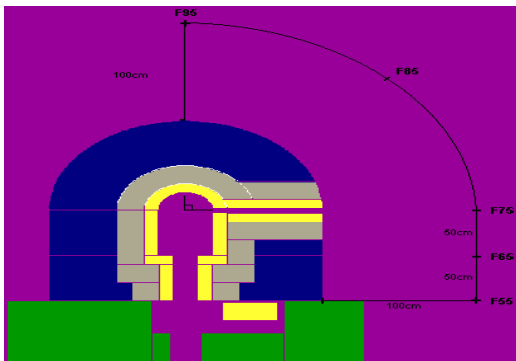
Figura 4. Corte de la simulación de blindaje radiológico, ubicando tally y configuración de colimación del haz difractado en 90°.
