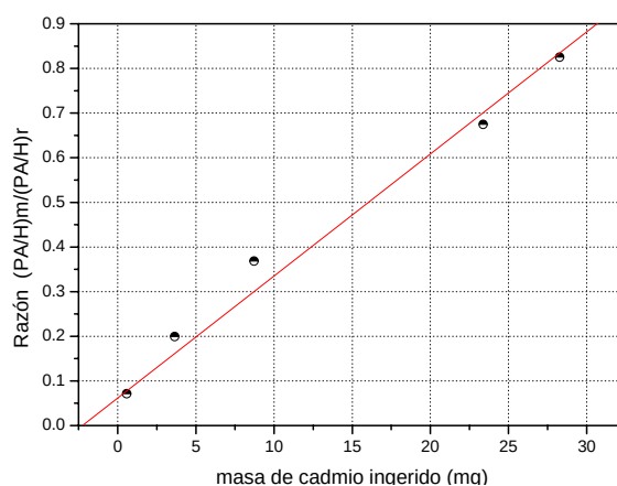
Figura 6. Razón de señales para muestra y referencia en función de cadmio incorporado, (\text{Cd}/\text{H})_m (\text{Cd}/\text{H})_r son la relación a la incorporación de cadmio en muestra biológica.
