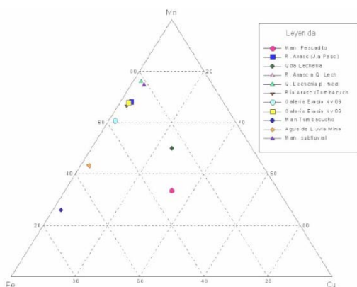
Figura 2. Diagrama Fe-Cu-Mn.
