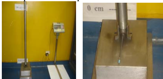
Figura 6. Sistema para ensayo de impacto y martillo sobre la cápsula del porta fuente.
