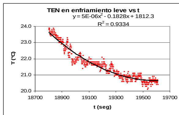
Figura 5. Etapa de enfriamiento leve (lapso de 17 minutos).
