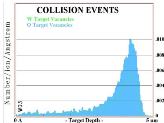
Figura 7. Distribución de las vacancias creadas por colisiones de las partícula \alpha en \text{WO}_3 .
