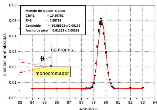
Figura 6. Ubicación angular de haz difractado, censado en la posición de la porta muestra.
