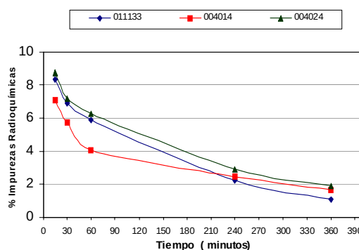
Gráfico 1. Estabilidad del ^{99m}\text{Tc} -MAA post-marcación, impurezas radioquímicas
