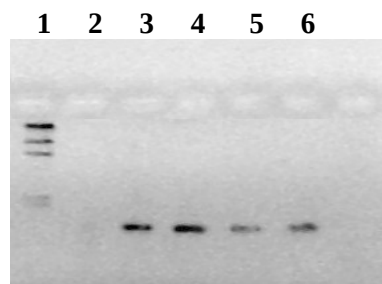
Figura 2. Electroforesis en gel de agarosa 1% de amplificados del 16S rRNA de microorganismos biooxidantes. Buffer TBE 0.5X, 40V, 40min. 1. Marcador \lambda /HindIII(50 ng/ul) 2. control negativo de reacción (sin muestra), 3. subcultivo de DAM Tamboraque, 4. cultivo de biorreactor, 5. L. ferrooxidans DSM 2705 T (control positivo), 6. A. ferrooxidans ATCC 19859 (control positivo).
