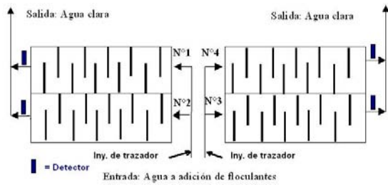
Figura 2: Arreglo experimental para la evaluación simultanea de las dos baterías de floculadores hidráulicos, mostrando los puntos de inyección y detección del radiotrazador.
