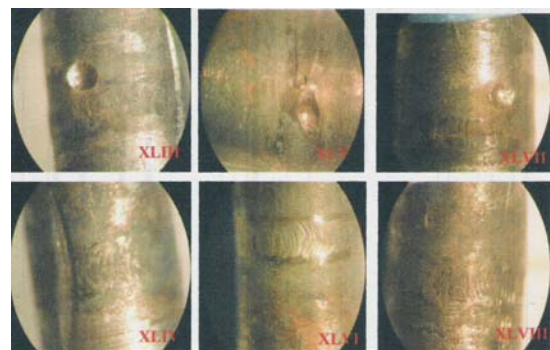
Figura 13. Ensayo de Punzado en la soldadura de los portafuentes.
