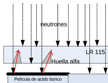
Figura 4. Esquema de ubicación de muestra borada y plástico detector frente al haz de neutrones.
