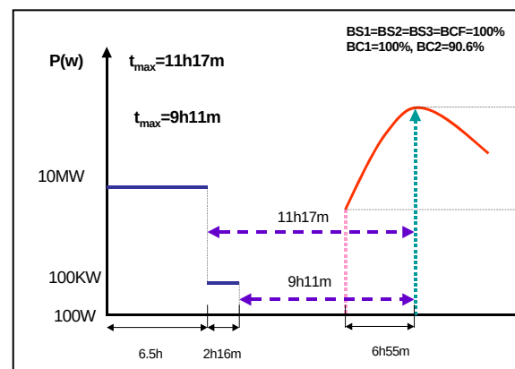
Figura 6. Esquema de la identificación del tiempo de máxima concentración con referencia a la bajada de 10 MW, 11horas y 17 minutos, mientras que si la referencia es la bajada de 100KW el tiempo es 9horas con 11 minutos.
