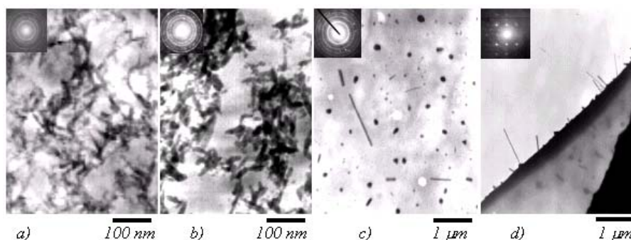
Figura 5. Micrografías MET que muestran la morfología del \text{TiO}_2 con su respectivo patrón de difracción de electrones obtenidos. a) 2; b) 6; c) 20 y d) 30 horas de peptización respectivamente.
