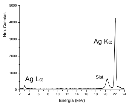
Figura 6. Espectro de fluorescencia de rayos X correspondiente a la muestra preparada a 700 °C
