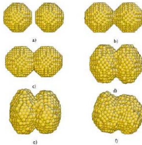
Figura 2. Evolución temporal del proceso de coalescencia a 300 K de dos NP de cobre con velocidad de impacto de 800 m/s: a) 0.32 ps, b) 0.96 ps, c) 1.60 ps, d) 2.88 ps, e) 3.84 ps, f) 8.64 ps. Para la visualización se utilizó el programa Atomeye [15]
