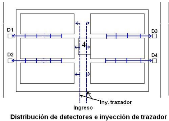
Figura 3. Arreglo experimental para la evaluación simultánea de los decantadores, mostrando los puntos de inyección y detección del radiotrazador.
