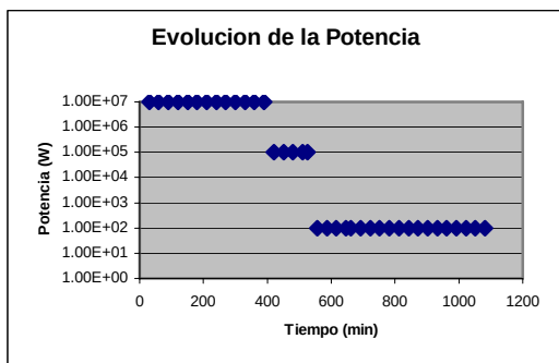
Figura 4. Registro de la evolución de la potencia del reactor durante la operación de determinación del tiempo de máxima concentración. Se presentan tres niveles 10 MW durante 5.5 horas, 100KW durante 2.1 horas y 100W hasta el fin de la experiencia.
