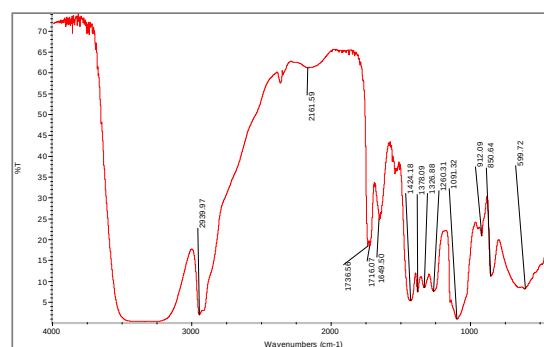
Figura 1. Espectro IR de la película de quitosano-PVA dopada con 1ppm de TiO 2 .
