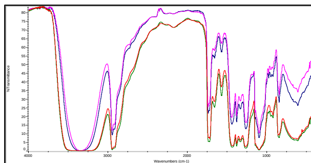
Figura 5. Espectros FT-IR de las películas de PVA (rojo) y PVA dopadas con 10ppm (verde), 100ppm (violeta) y 1000ppm (azul) de \text{TiO}_2 .
