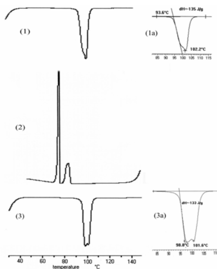
Figura 3. Termograma del 2-pentadecilbenzimidazol. (1) Primer proceso de calentamiento (1a) Ampliación de la endoterma del primer proceso. (2) Proceso de enfriamiento (3) Segundo proceso de calentamiento (3a) Ampliación de la endoterma en el segundo proceso de calentamiento.
