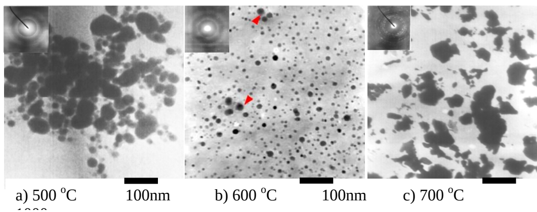
Figura 3. Micrografías MET de nanopartículas basados en Ag con sus respectivos patrones de difracción de electrones (esquina superior izquierda) obtenidos a las temperaturas indicadas.
