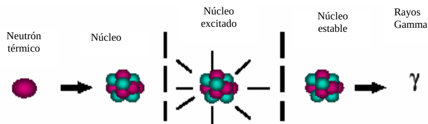
Figura 1. Secuencia de producción de los fotones gamma inmediatos.
