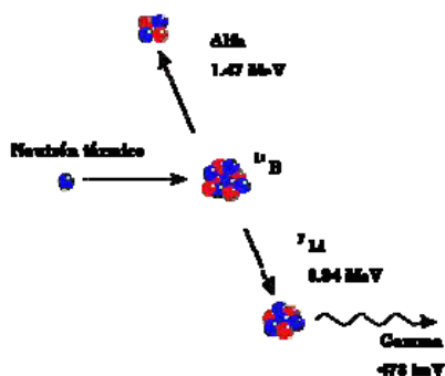
Figura 2. Interacción neutrónica en un átomo de boro.
