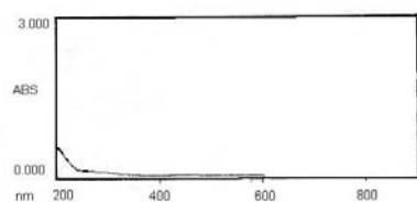
Gráfico 7. Espectro UV-VIS de Agua de remojo de Aloe vera , en trozos luego de 75 horas.
