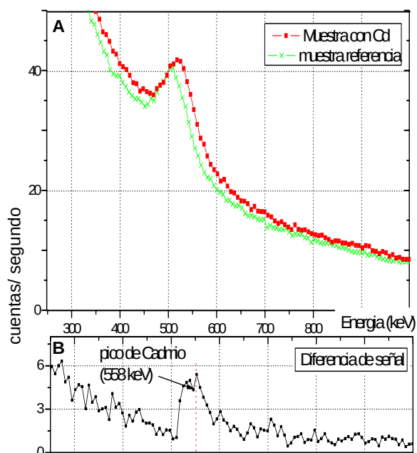
Figura 4. A: Espectro gamma de muestra biológica con \text{Cl}_2\text{Cd} y muestra biológica de referencia, tiempo de colección de espectro 300s, B: Diferencia de señales se nota el pico de cadmio (558.7 keV)
