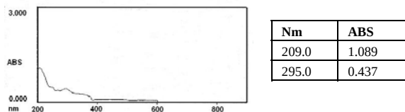
Gráfico 4. Espectro de Agua de remojo de hojas enteras de Aloe vera luego de 75 horas.
