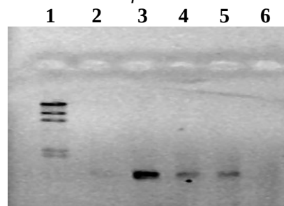
Figura 3. Electroforesis en gel de agarosa 1% de amplificados del 16S rRNA con primers pLepf y pLepr. Buffer TBE 0.5X, 40V, 50min. 1. Marcador \lambda /HindIII (50 ng/ul), 2. A. ferrooxidans ATCC 19859 (control negativo), 3. L. ferrooxidans DSM 2705 T (control positivo), 4. cultivo de biorreactor, 5. cultivo de DAM Tamboraque, 6. control negativo de reacción (sin muestra)
