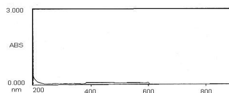
Gráfico 1. Espectro de Agua Destilada – Blanco.
