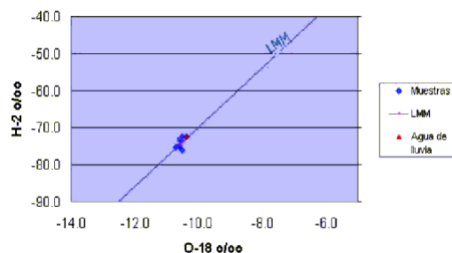
Figura 3. Diagrama Oxígeno-18 - Deuterio.
