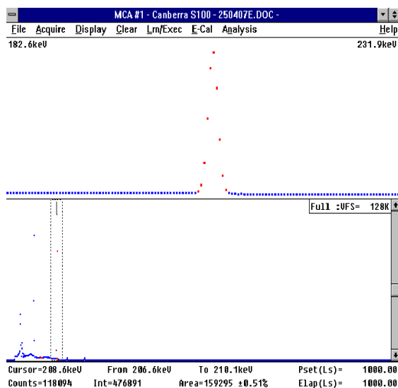
Figura 1. Pico característico del espectro gamma de Lutecio 177, obtenido a partir de un blanco enriquecido.
