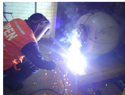
Figura 7. Fijación de cabezal a base metálica.
