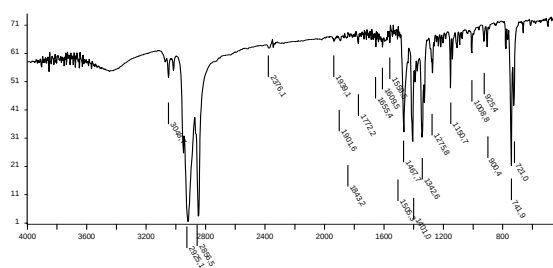
Figura 1. Espectro infrarrojo del 1,1'-bis(octadecil)-2,2'-bibenzimidazol.
