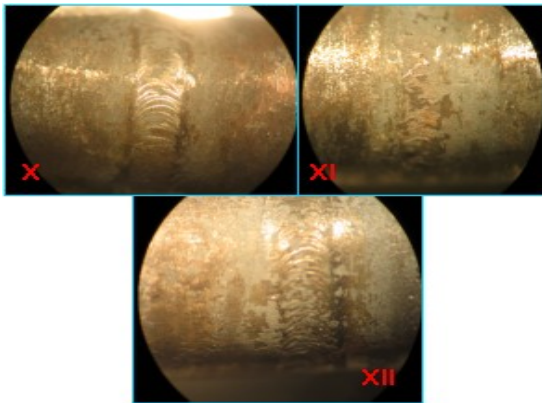
Figura 11. Unión soldada porta fuente-cápsula después de ensayos de temperatura.
